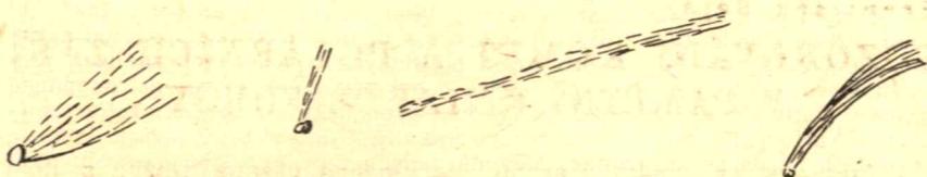
Kresby komet z let 1811, 1819, 1843 a 1858, pozorovaných V. Fuksou ve Střebčeticích.
