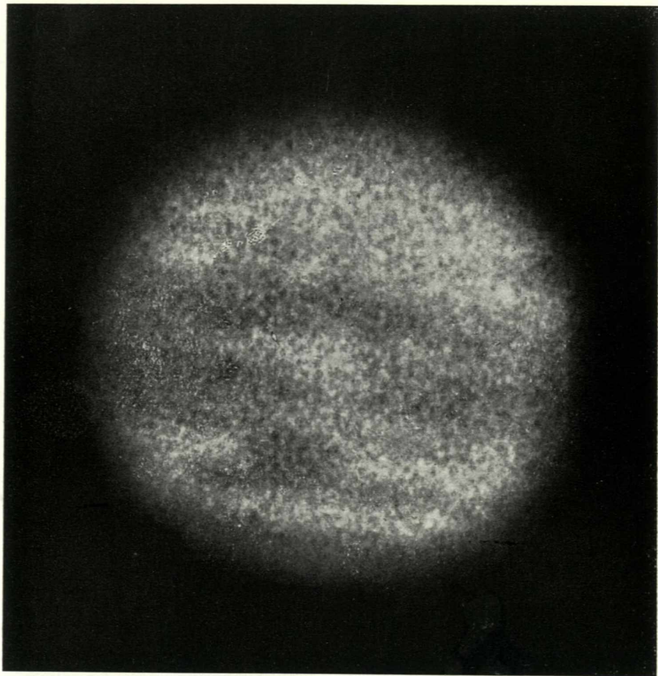
Fotografie Jupitera, získaná na lidové hvězdárně v Prostějově 10. prosince 1964 v 19 hod. 25 min. reflektorem o průměru 330 mm, ekvivalentní ohnisková vzdálenost 20 m.
