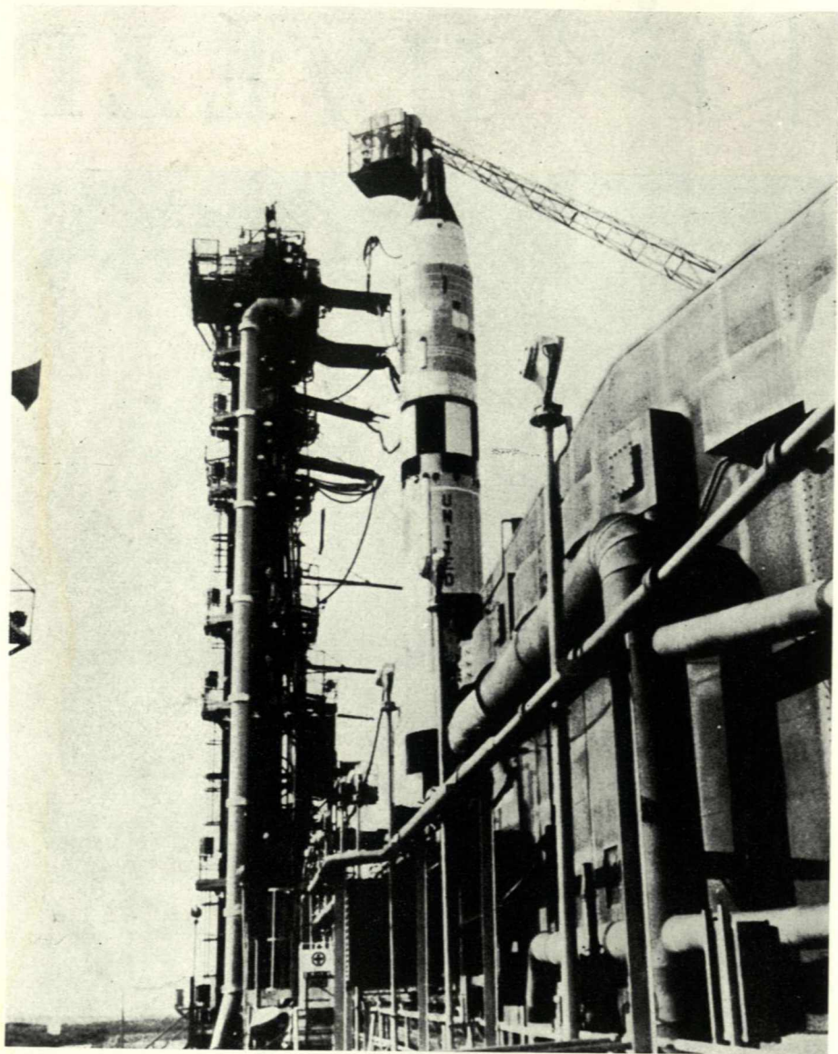
Dvoustupňová raketa Titan 2 s kosmickou loďí Gemini 5 (NASA). — Na první straně obálky je část rovníkové oblasti odvrácené polokoule Měsíce v okolí Mare Orientalis, fotografovaná stanicí Zond 3 (TASS).
